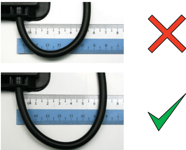
Abb. 8: Beispiel für falsche und richtige Biegung eines Kabels beim Verlassen der Junction Box.
