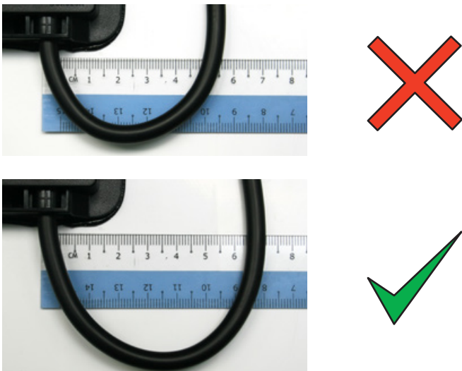
Fig. 8: Ejemplos de flexión de cable incorrecta y correcta saliendo de la caja de conexiones
