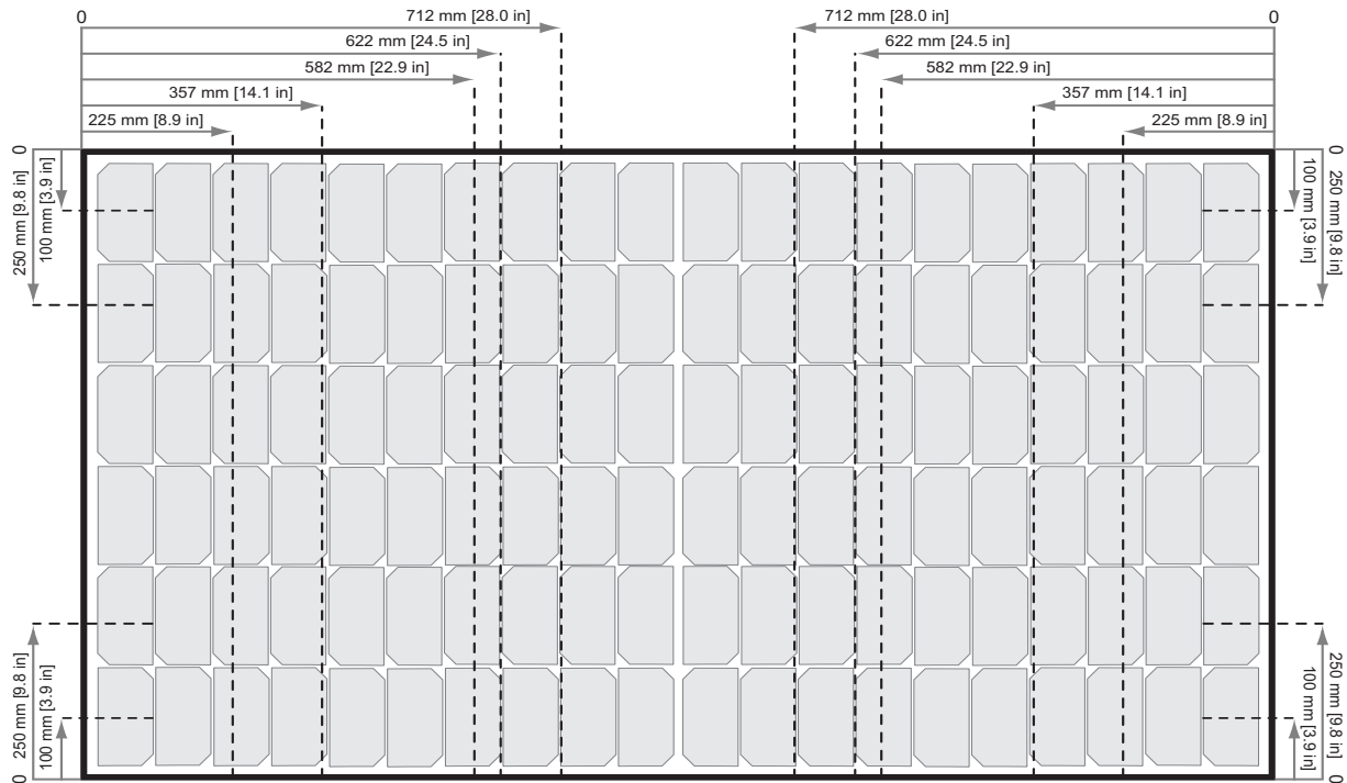
Fig. 11: Fijación de los paneles REC N-Peak 2 con ralles cortos
