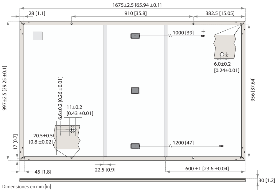
Fig. 22: Dimensiones del panel: Serie REC N-Peak Black
