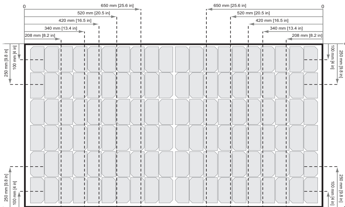
Fig. 8: Fijación de los paneles REC N-Peak con raíles cortos
