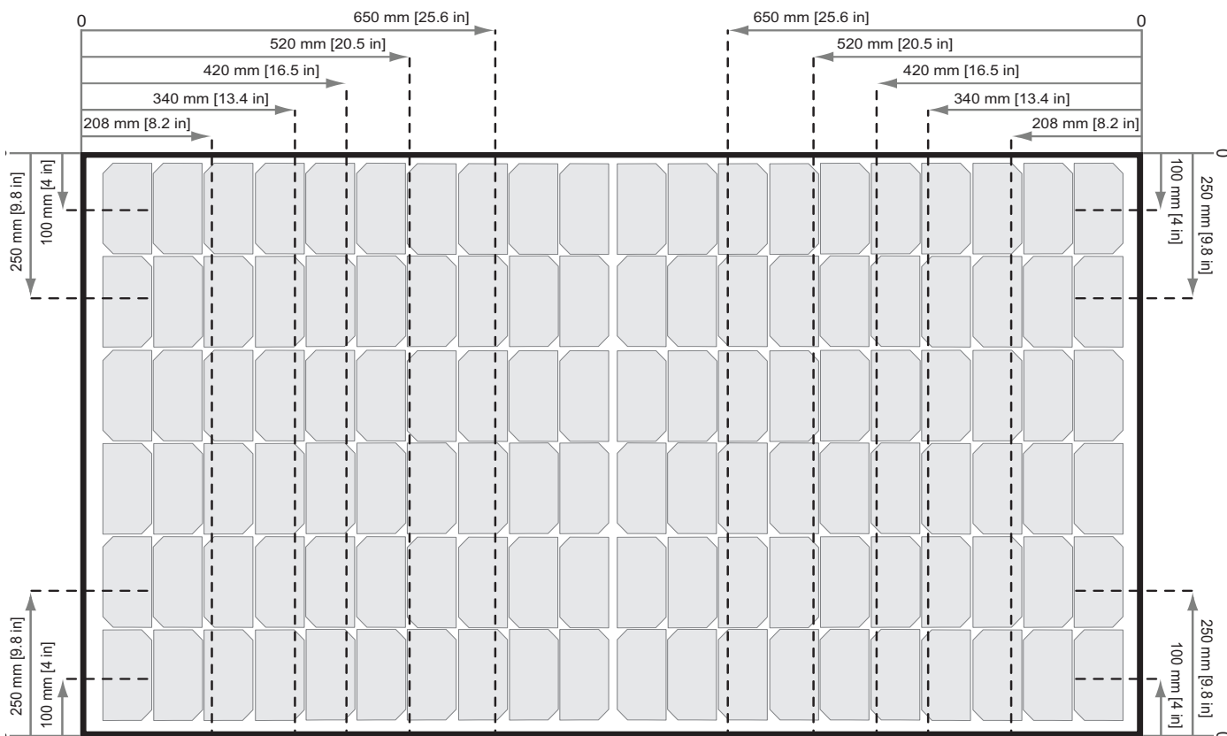
Fig. 6: Fijación de paneles N-Peak con raíles paralelos al lado corto del panel
