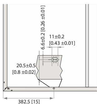
Fig. 12: Orificios de montaje: Paneles REC de 60 células
