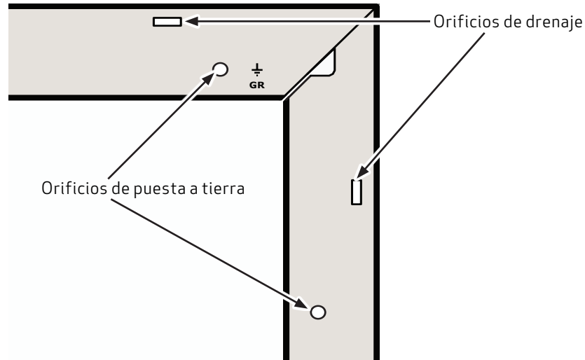
Fig. 16: Orificios de drenaje y puesta a tierra
