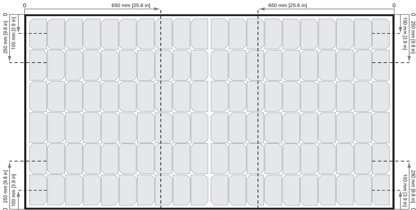
Fig. 10: Fijación de paneles N-Peak 2 con raíles paralelos al lado largo del panel
