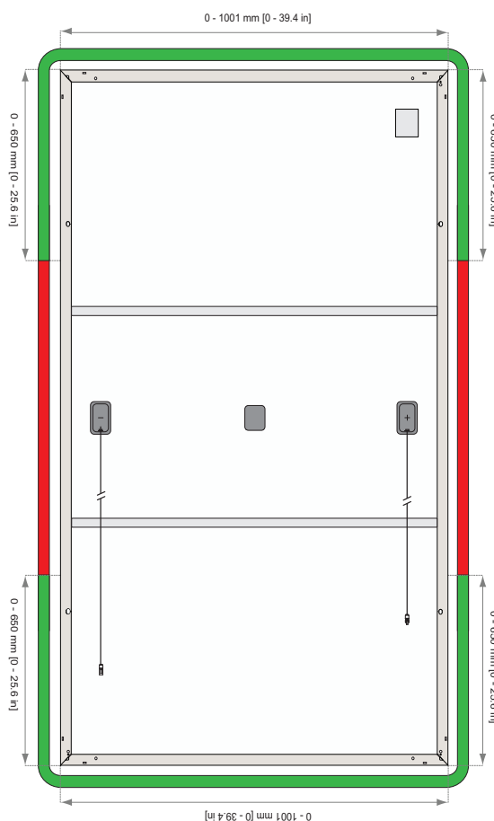
Fig. 26: Zonas de instalación de dispositivos MLPE en los paneles REC de 72 células
