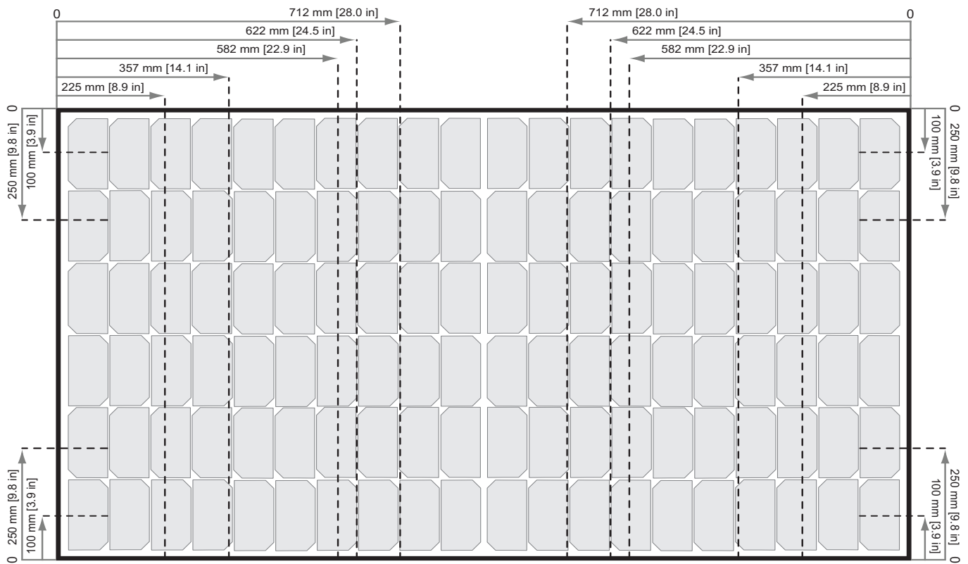
Fig. 9: Fijación de paneles N-Peak 2 con raíles paralelos al lado corto del panel
