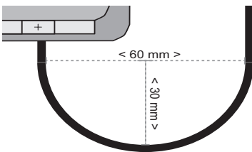
Fig. 17: Radio de flexión mínimo del cable
