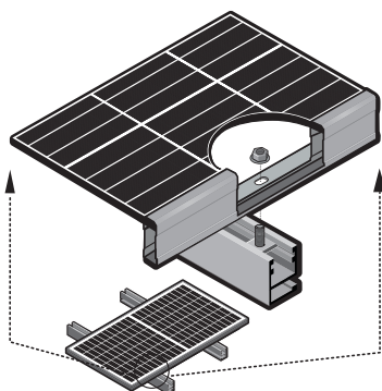
Fig. 15: Ejemplo de instalación de los orificios de montaje
