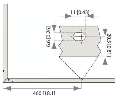
Fig. 13: Orificios de montaje: Paneles REC de 72 células
