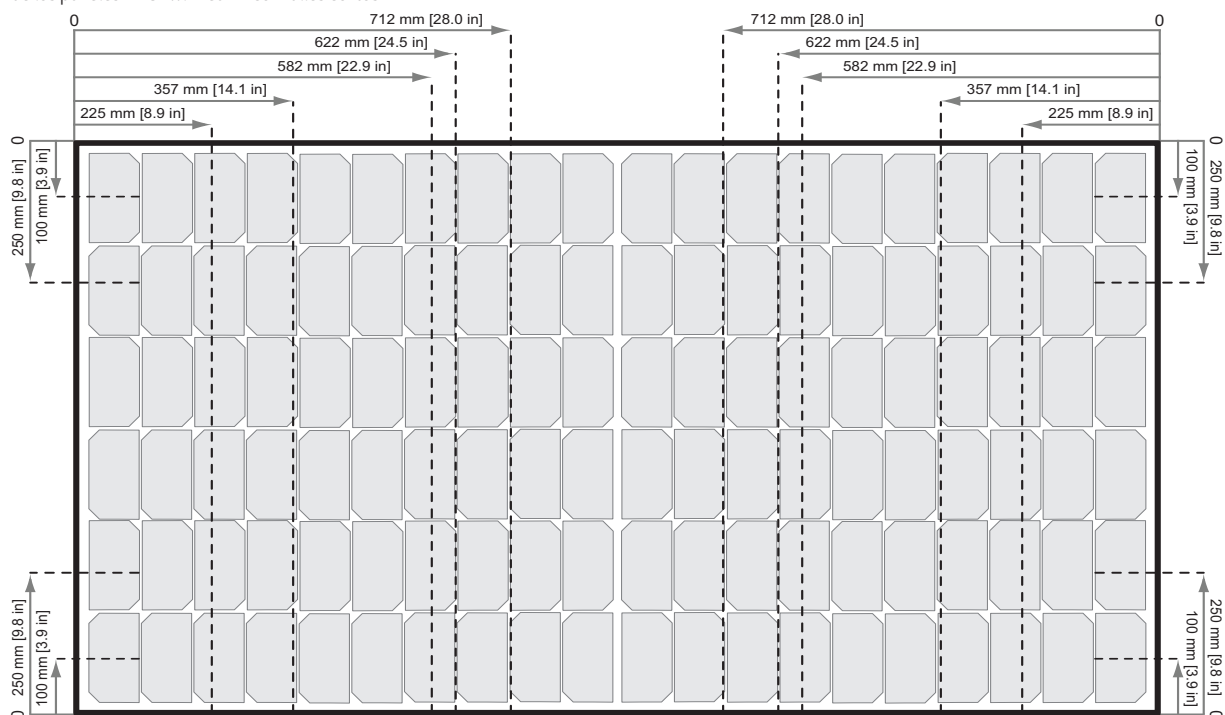
Fig. 5: Fijación de los paneles REC TwinPeak 4 con raíles cortos
