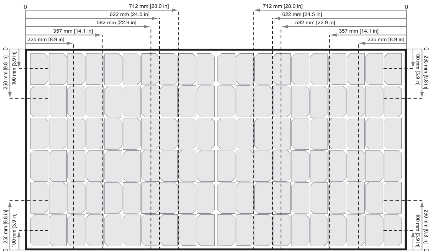
Fig. 3: Fijación de paneles TwinPeak 4 con raíles paralelos al lado corto del panel
