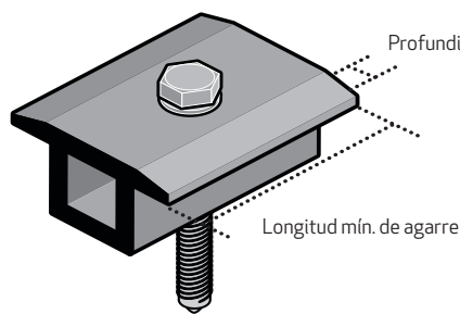
Fig. 1: Especificaciones de las abrazaderas
