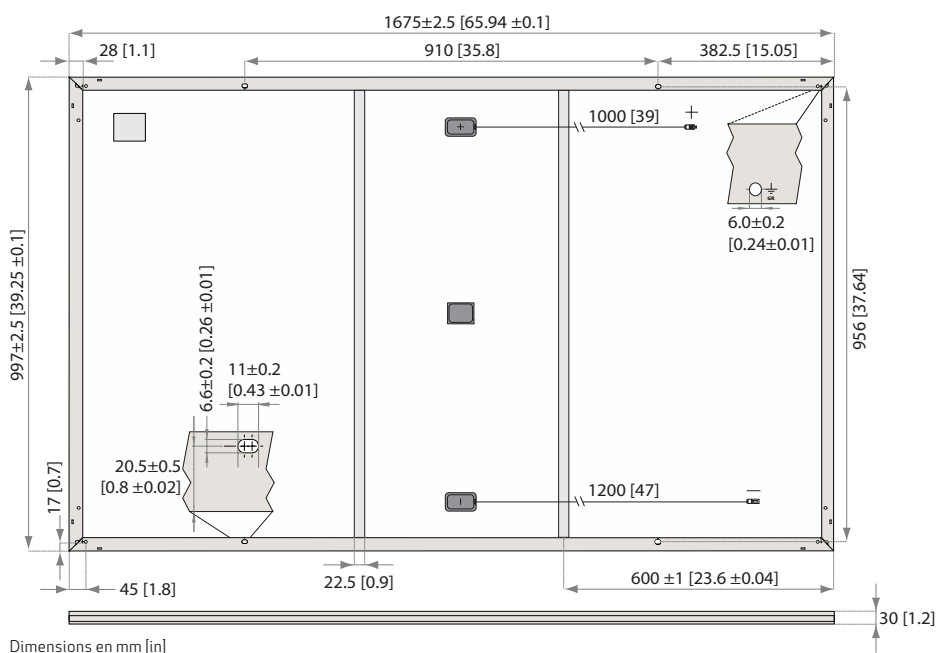
Fig. 22: Dimensions du panneau: REC N-Peak Black Série
