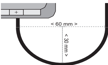
Fig. 17 : Rayon minimal de courbure du câble
