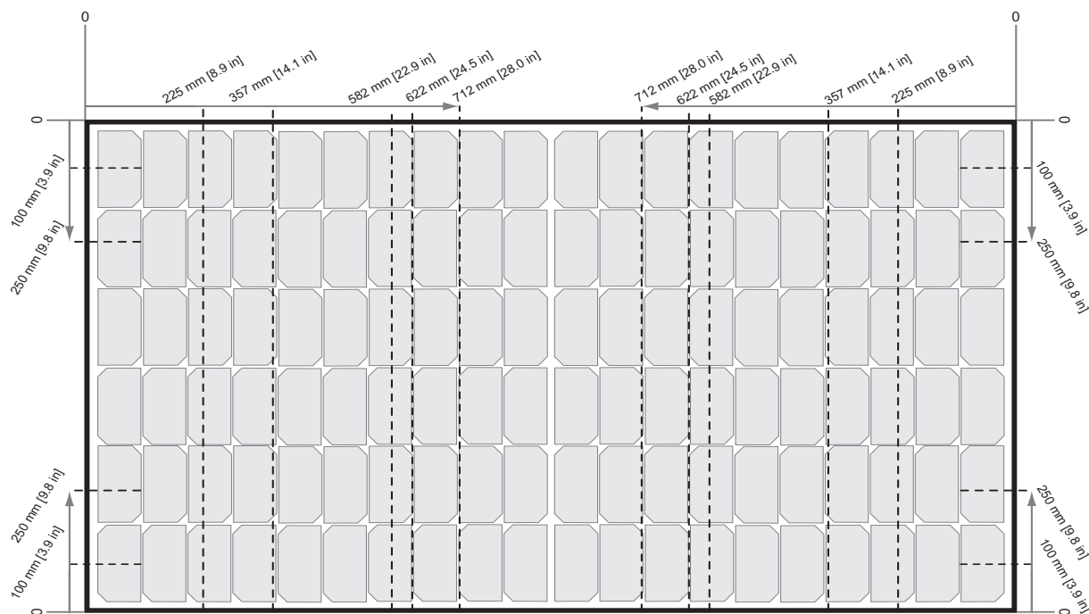
図5: 短いレールを使用したTwinPeak 4モジュールのクランプ
