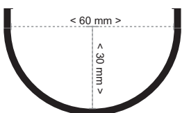
図14: ケーブルの最小曲げ半径
