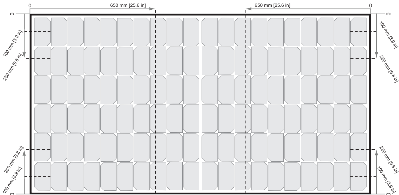
図4: TwinPeak 4モジュールでレールをモジュールの長辺に平行にしたクランプ
