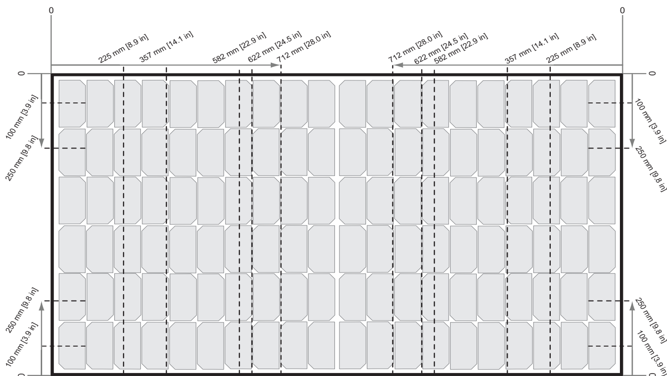
図3: TwinPeak 4モジュールでレールをモジュールの短辺に平行にしたクランプ
