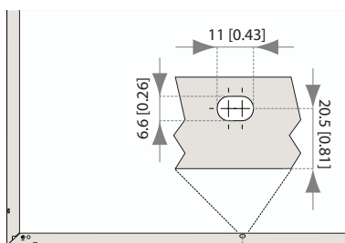
図9:取り付け穴
