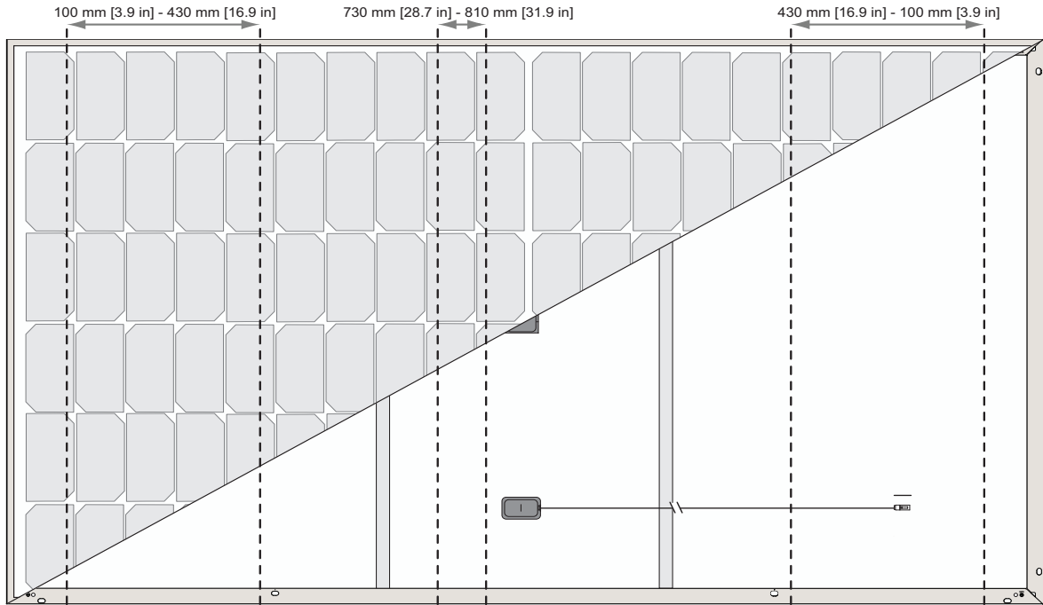
図12:6点留めのクランピングゾーン
