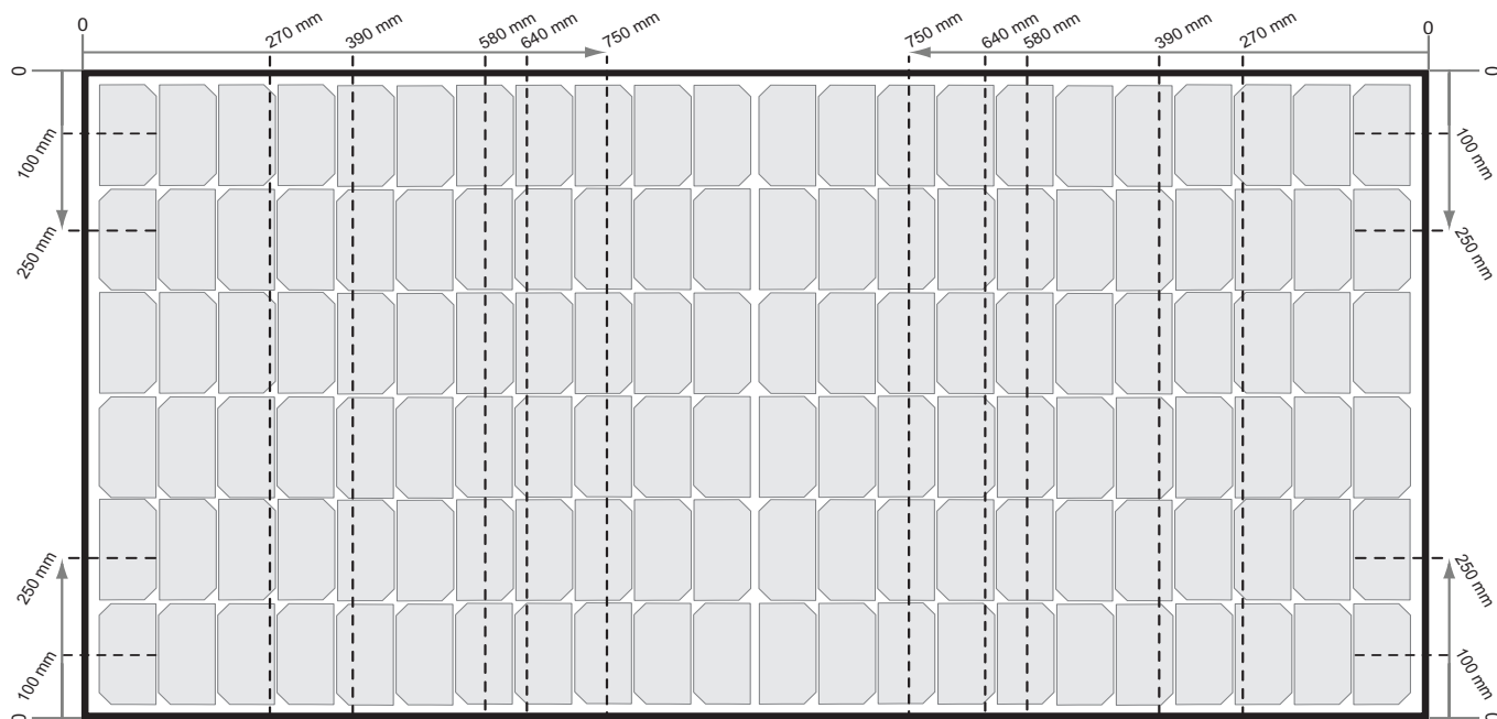
図6: TwinPeak 5モジュールでレールをモジュールの短辺に平行にしたクランプ
