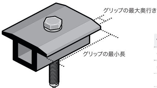
図1: クランプの仕様
