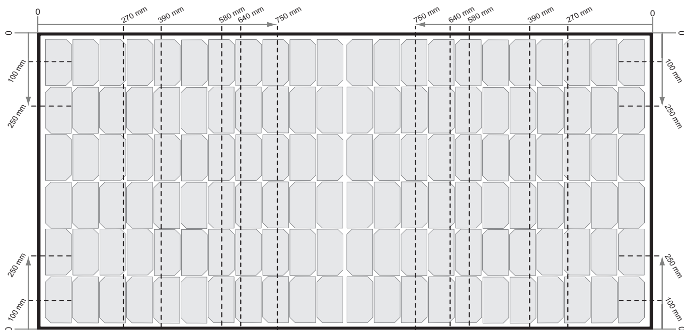
図8: 短いレールを使用したTwinPeak 5モジュールのクランプ
