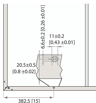
Afb. 12: Montagegaten: REC-panels met 60 cellen
