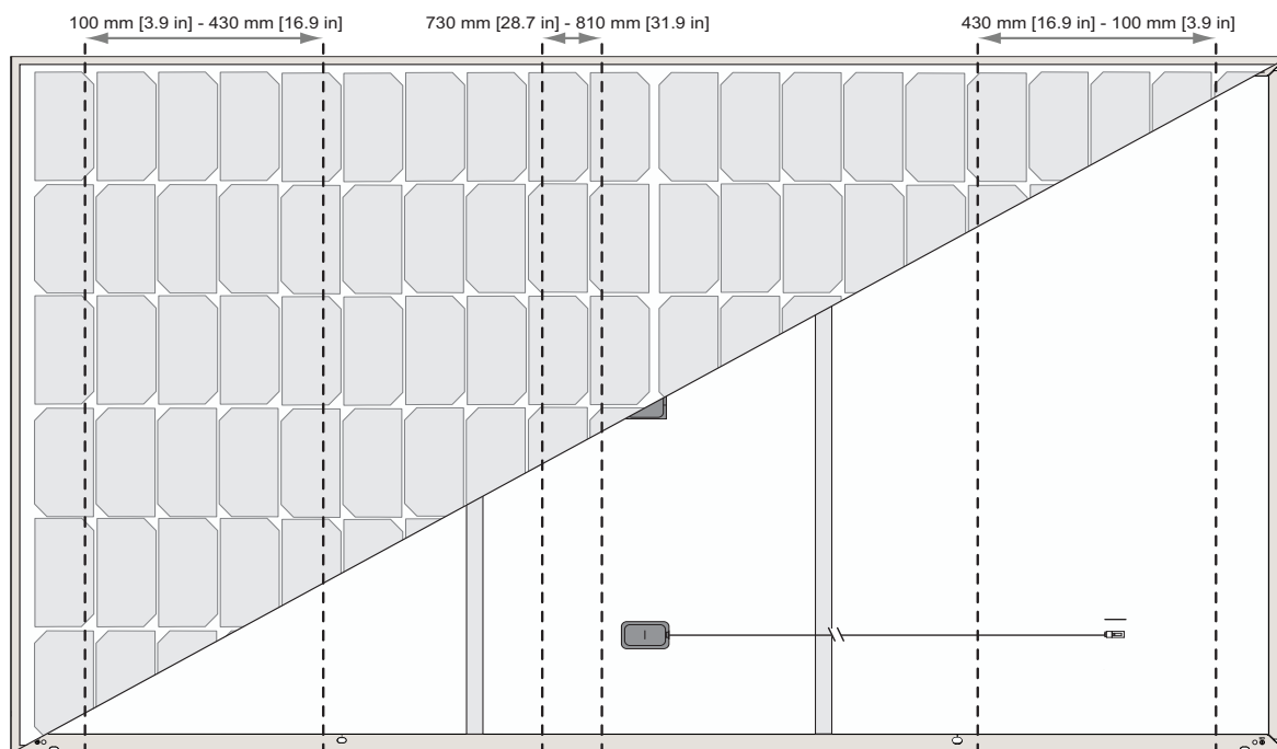
Afb. 27: Zes-punts montage klemzones
