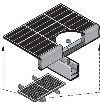
Afb. 15: Installatievoorbeeld met montagegaten
