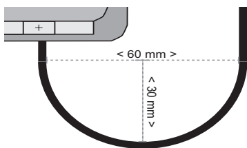
Afb. 17: Minimale buigstraal van kabel
