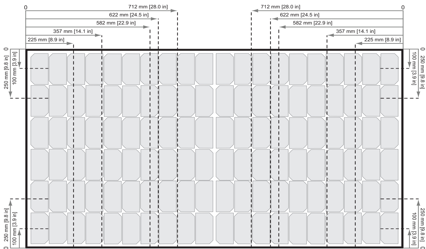
Afb. 9: Vastzetten van N-Peak 2-paneleen op rails evenwijdig met de korte zijde van de module
