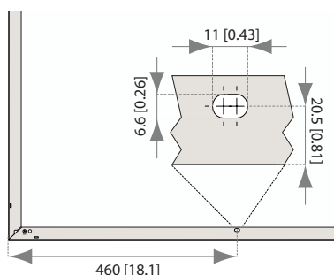
Afb. 13: Montagegaten: REC-panels met 72 cellen
