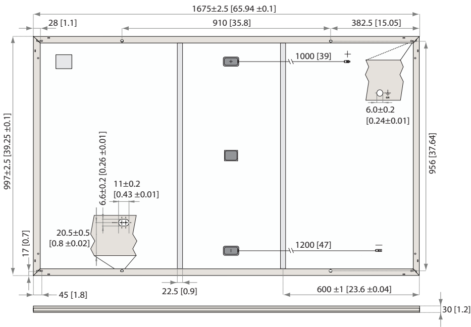
Afb. 21: Paneel afmetingen: REC N-Peak-serie
