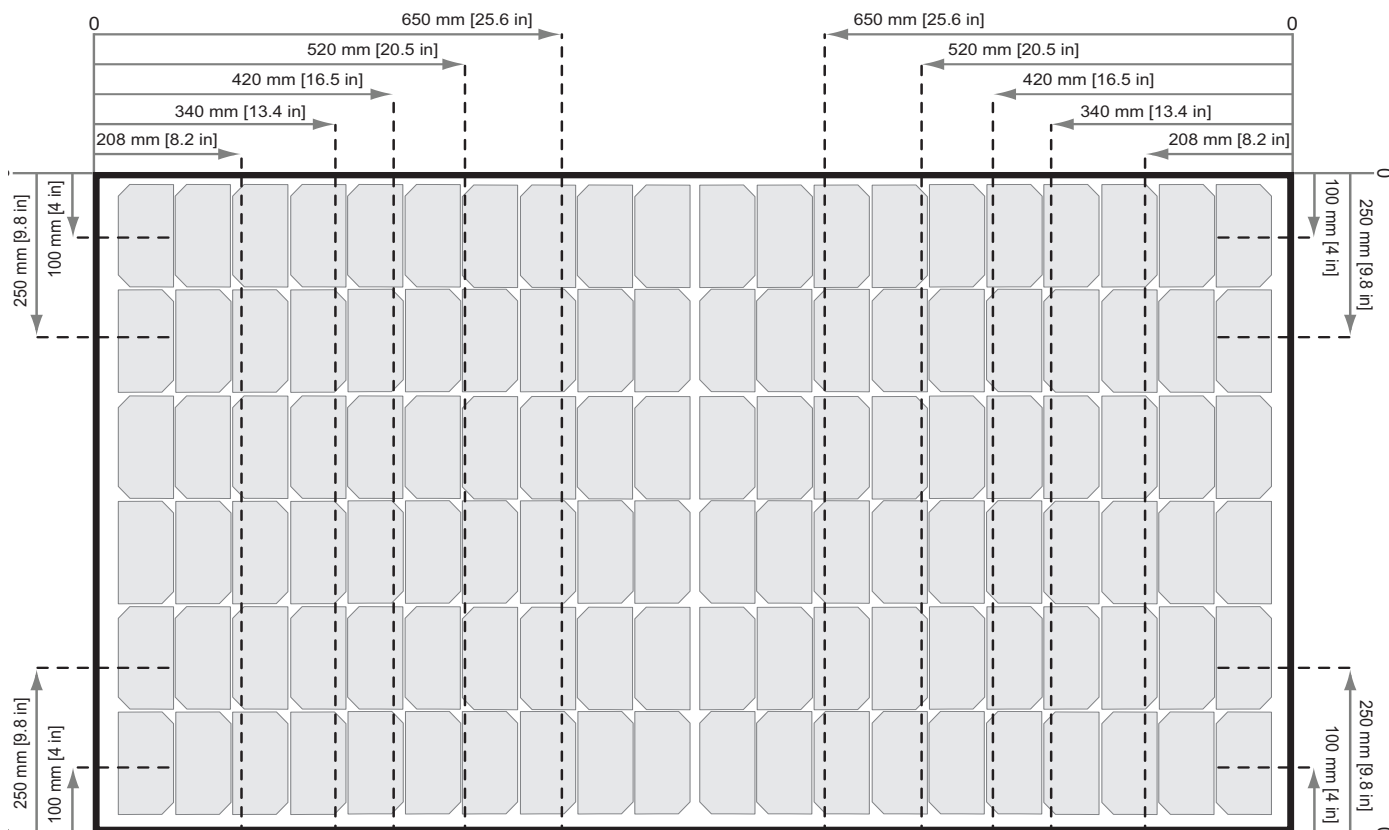
Afb. 6: Vastzetten van N-Peak-panels op rails evenwijdig met de korte zijde van de module
