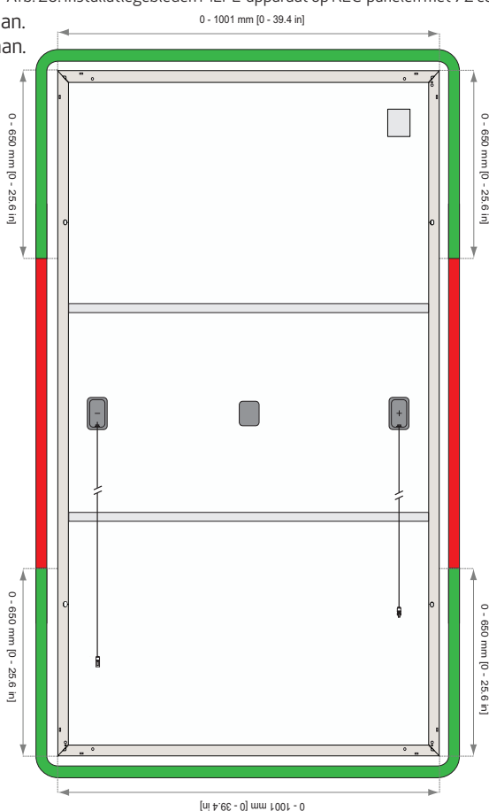
Afb. 26: Installatiegebieden MLPE-apparaat op REC-panels met 72 cellen
