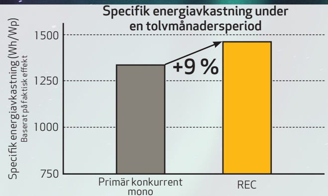
Källa: Jämförande test av utomhusmodul, SERIS, Singapore, 2019
